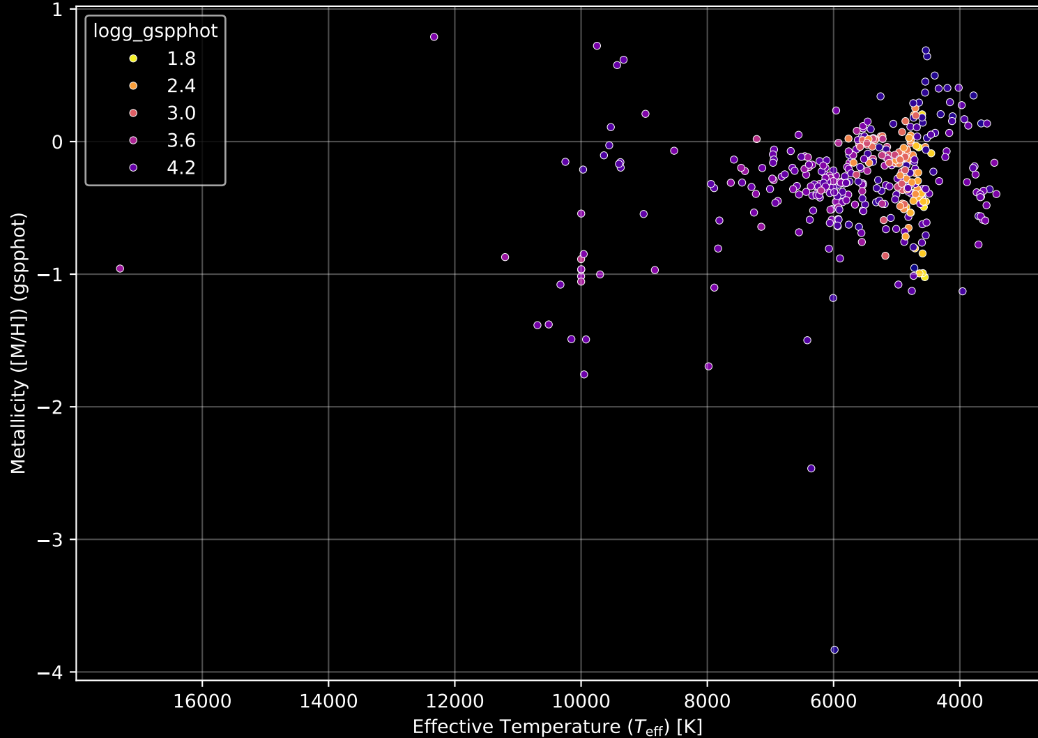
APOGEE DR17 Field: [ORIONOB1AB-E] Stellar Population Parameters (n= 412)
